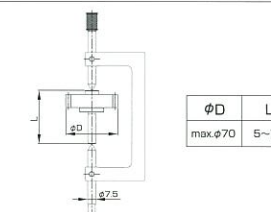
関係寸法図 Related drawing
