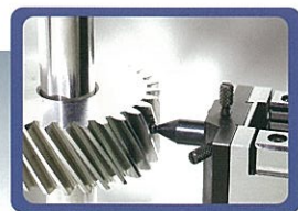
CS-251型測定機構 MODEL: CS-251 Measuring mechanism
