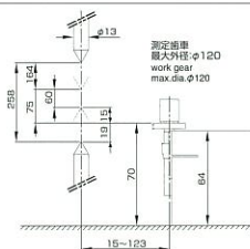
関係寸法図 Related drawing
