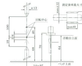
関係寸法図 Related drawing
